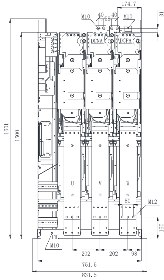
图 3-4 正视图
