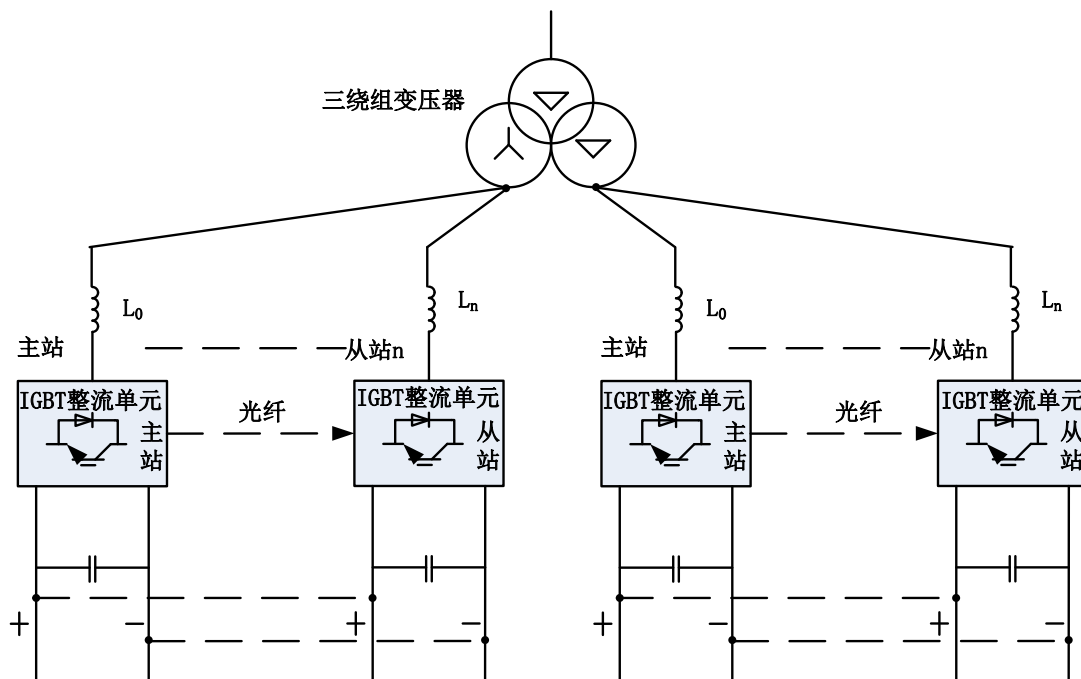
图 2-15 12 脉冲并联方式
