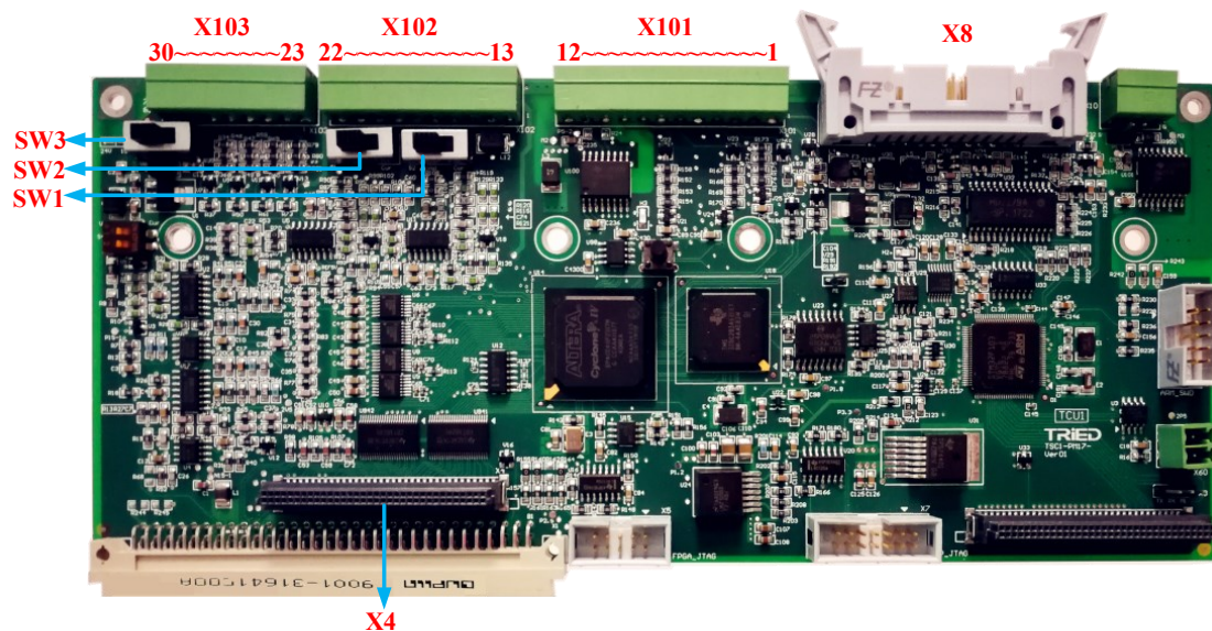
图 4-5 Tried 控制板
