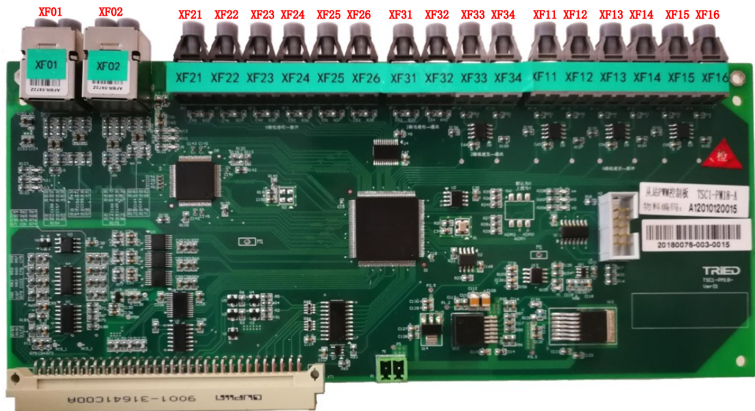
图 4-4 PWM 板
