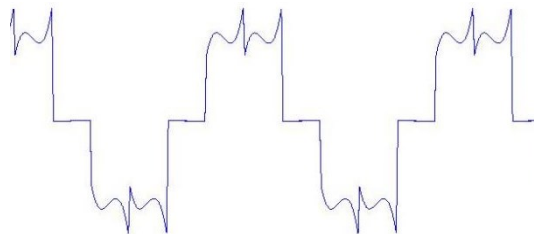
图 2-3 回馈电流波形
