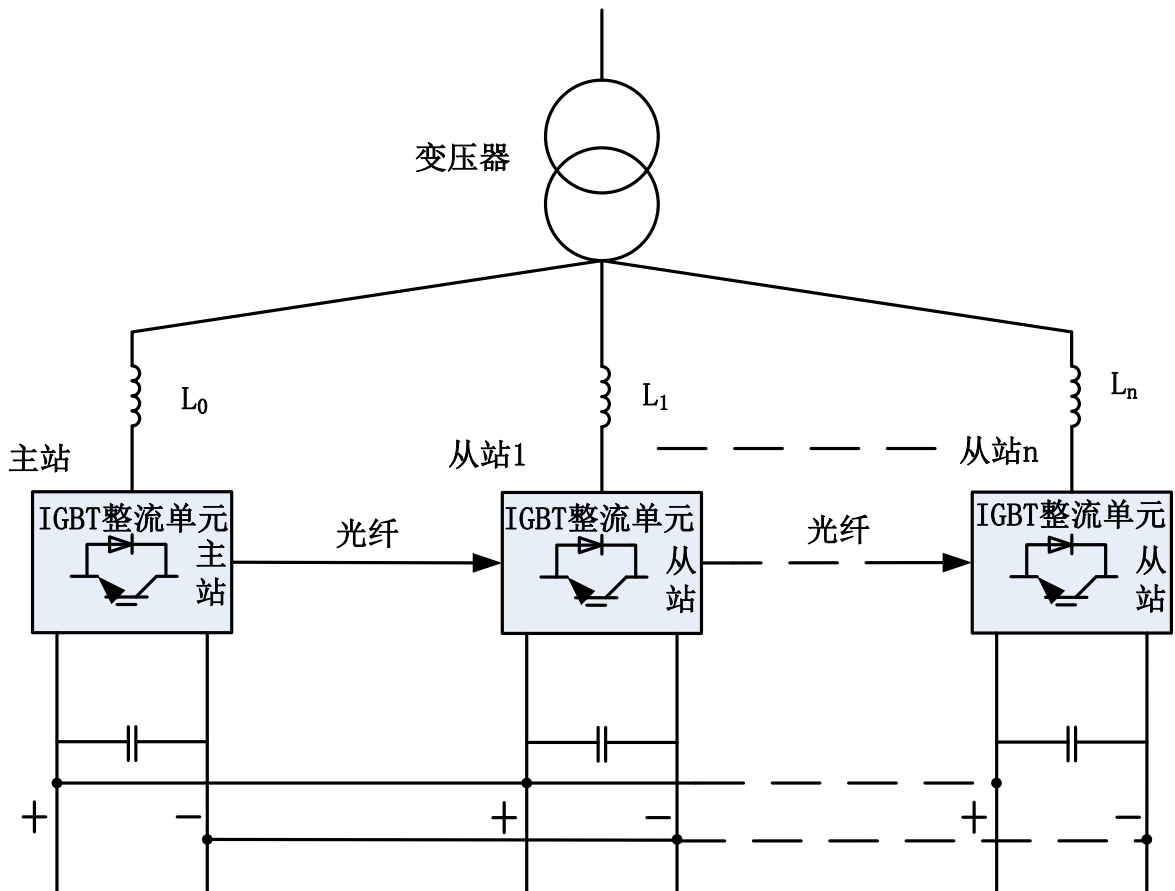
图 2-14 6 脉冲并联方式
