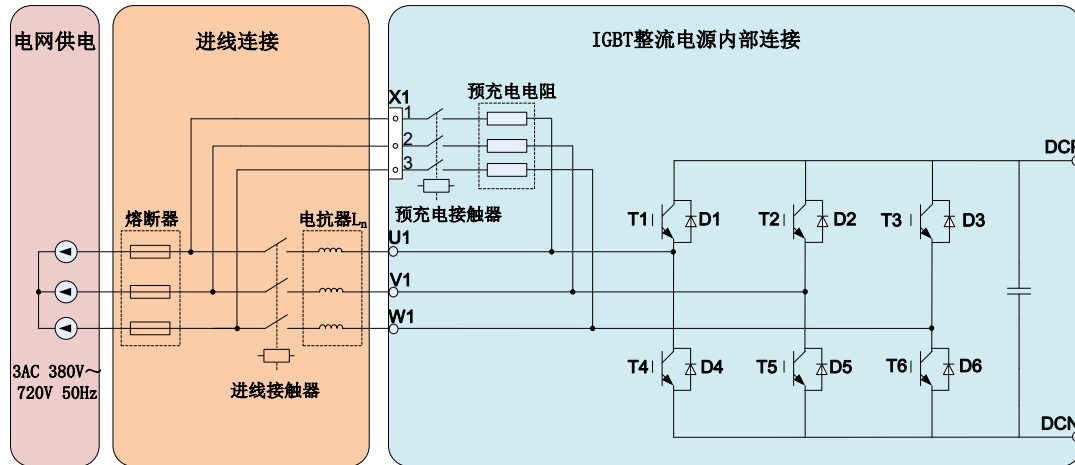
图 2-4 由 D 型 IGBT 整流电源组成的整流系统
