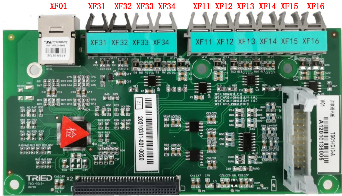
图 4-6 高速通讯板
