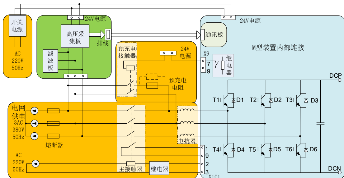
图 2-9 M 型 IGBT 整流电源组成的整流系统
