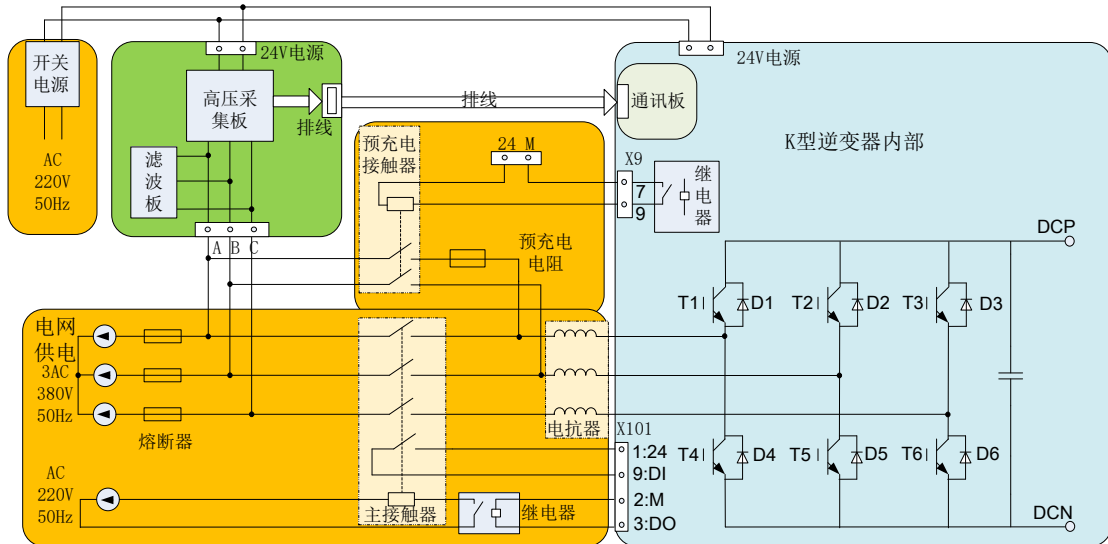
图 2-6 K 型 IGBT 整流电源组成的整流系统
