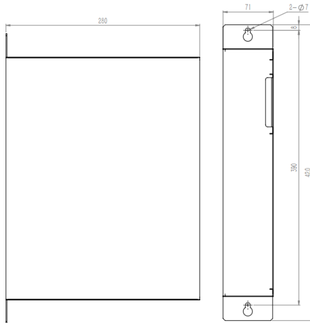
图 2-8 检测单元盒尺寸图
