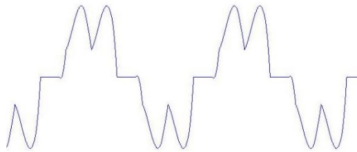
图 2-1 整流状态时交流电流波形
