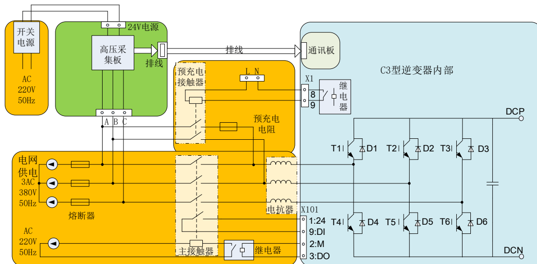
图 2-5 由 C3 型 IGBT 整流电源组成的整流系统
