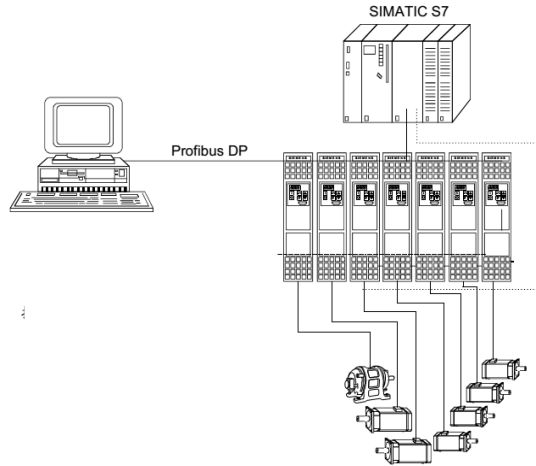
图 8.1 通讯
