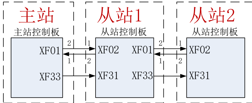
图 4-8 三台 IGBT 整流电源并联光纤连接图
