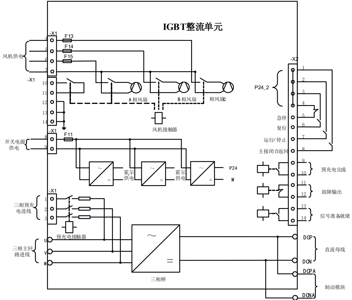
图 4-3 D 型 IGBT 整流电源内部结构
