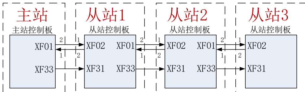
图 4-9 四台 IGBT 整流电源并联光纤连接图
